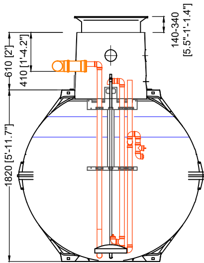
Querschnitt Belebungs- section SBR reactor
