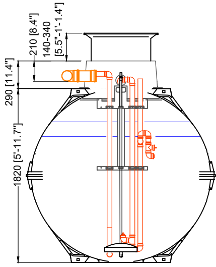
Querschnitt Belebungs section SBR reactor
