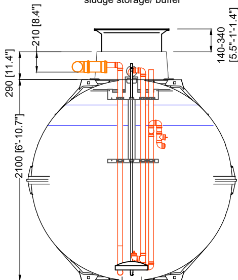
Querschnitt Belebung section SBR reactor
