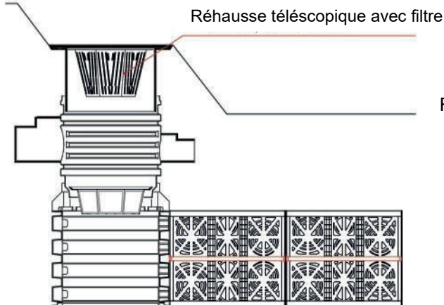
Regard de débordement
