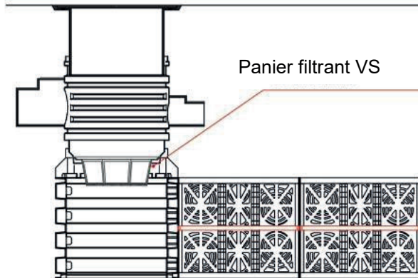
Regard de filtration
