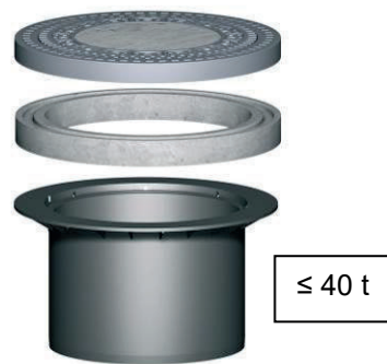
Rehausse télescopique pour couvercle en béton ou en fonte
