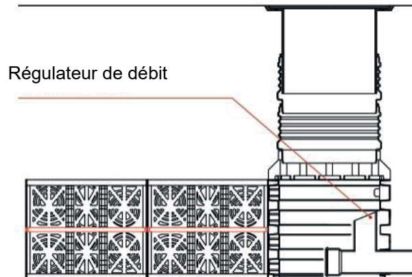
Regard à débit régulé
