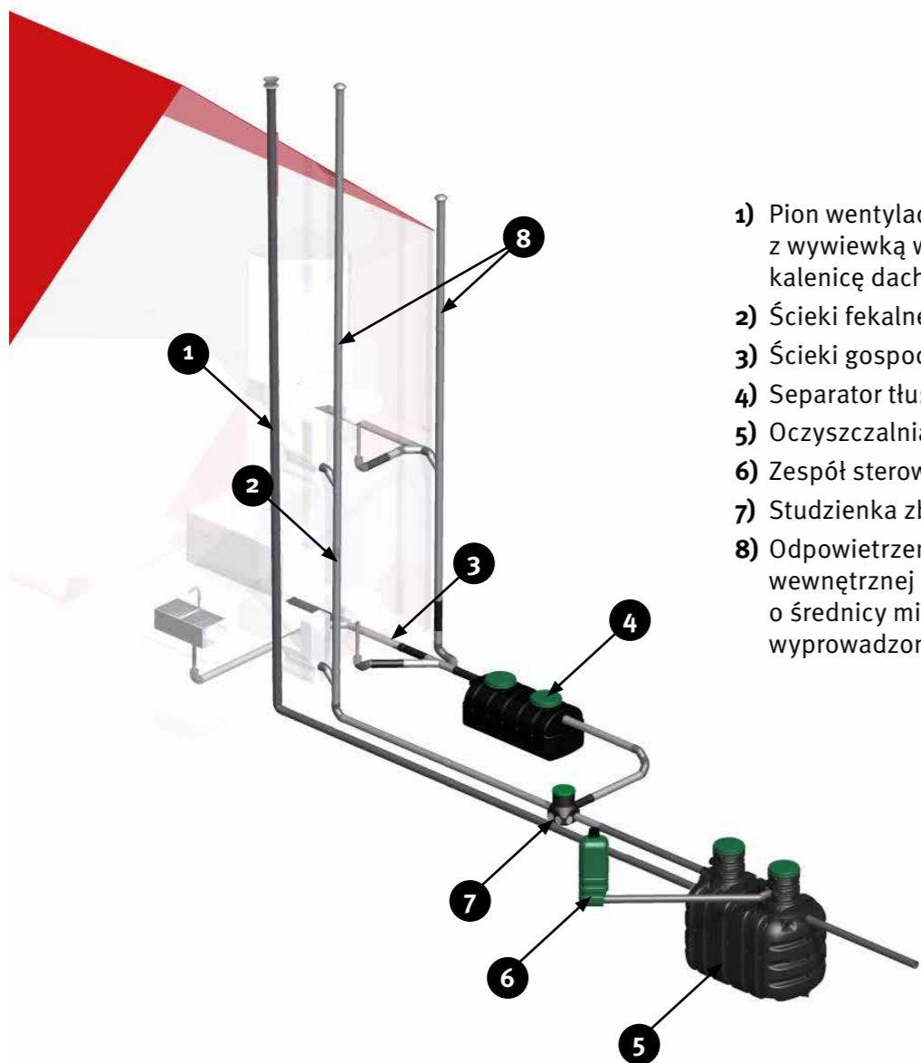
Rysunek 3. Montaż oczyszczalni easybio.
