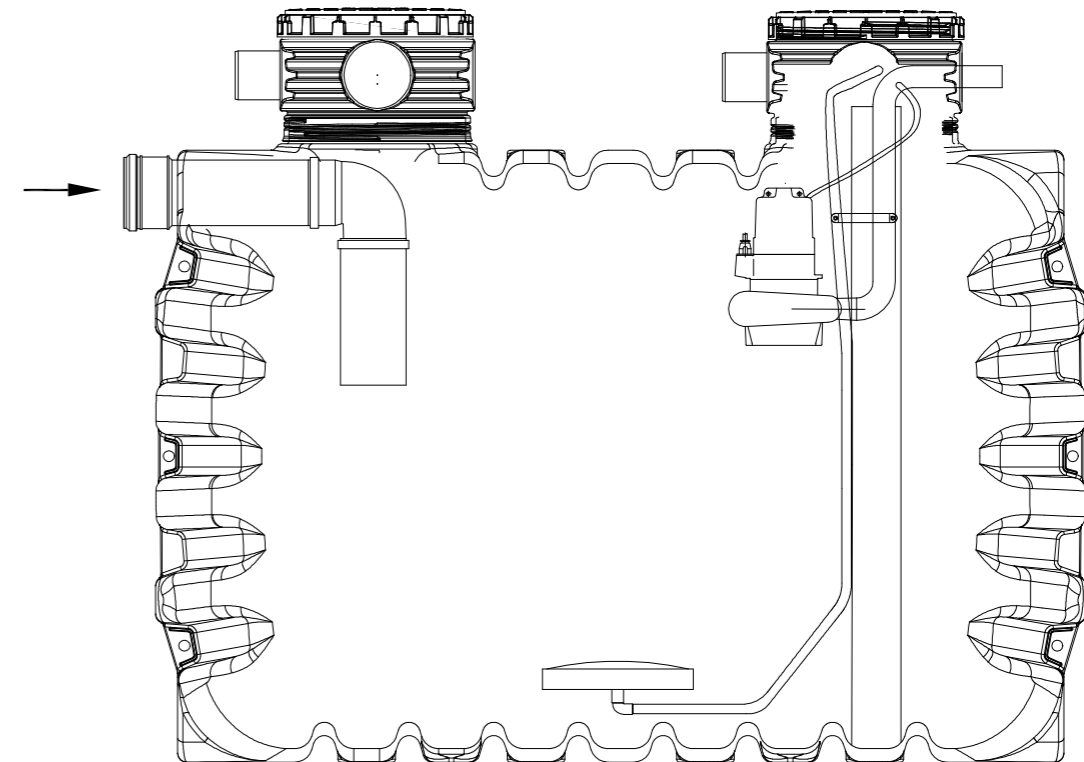
Rysunek 1. Przekrój oczyszczalni easybio z IPS.
