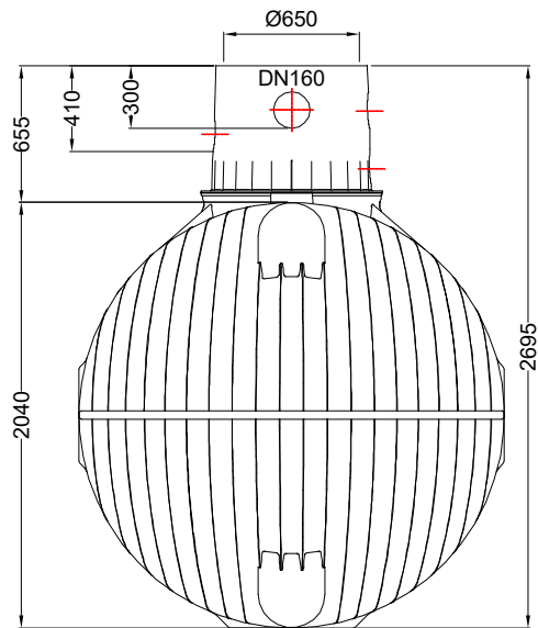
CARAT XL 8500 I zbiornik podziemny
